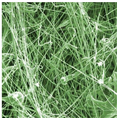
Abb. 4: Keramikfasern, Bildbreite 10 µm
