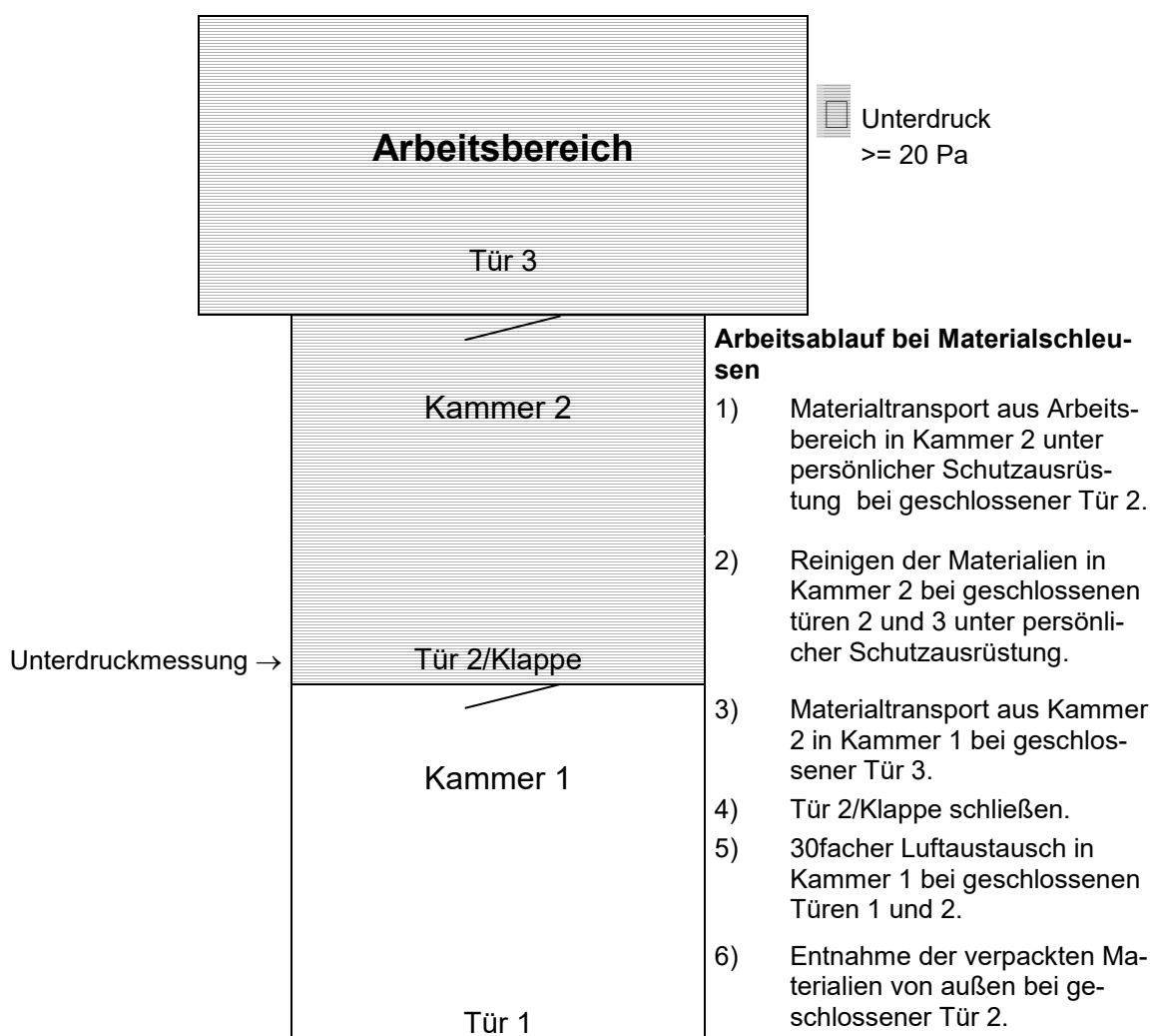
Abb. 2: Materialschleuse (Prinzipiskizze)
